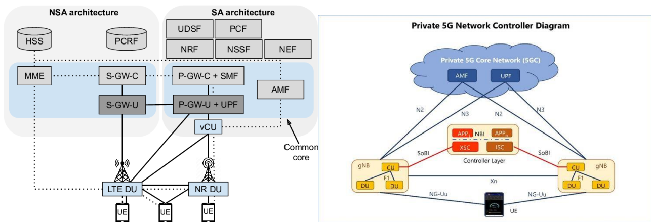
სურ. 1. „დამოუკიდებელი არქიტექტურული“ კონფიგურაცია SA (standalone architecture) და „არა დამოუკიდებელი“ NSA (non-standalone architecture) ქსელის არქიტექტურა, 5G ქსელის
